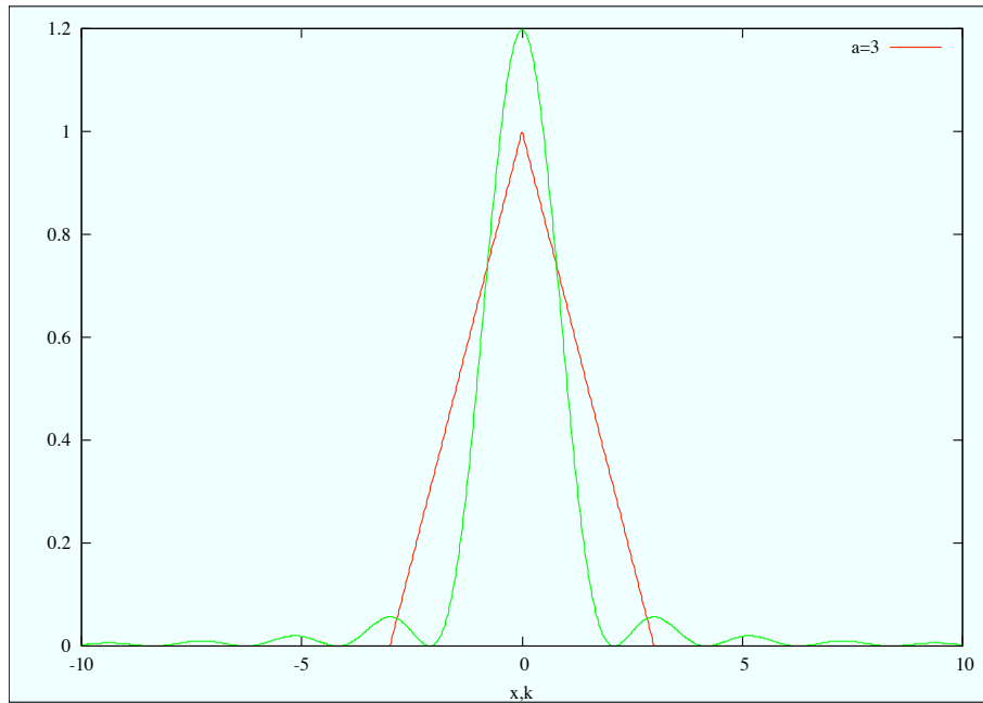
Figura 8: La funzione relativa all'esempio 2 e la sua trasformata di Fourier di scala. Facendo l'antitrasformata per a = 1 e x = 0 si ha:
