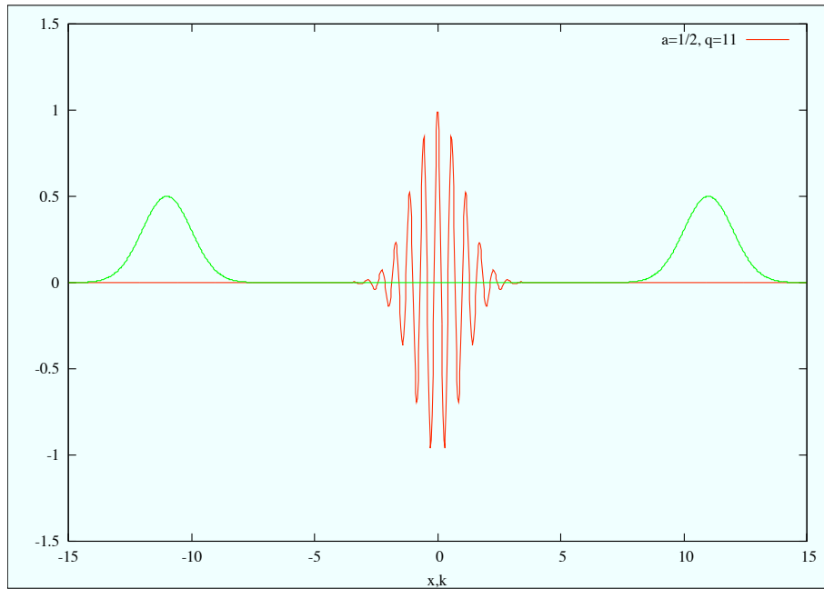
Figura 9: La funzione wave-packet e la sua trasformata di Fourier
