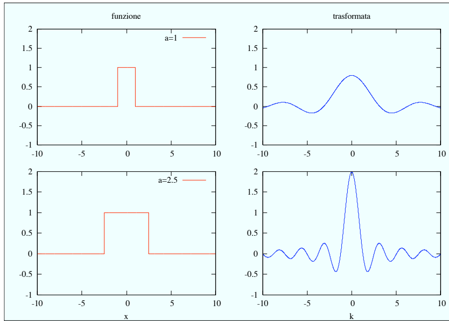
Figura 7: Trasformata di Fourier per la funzione top-hat per due valori di a .
