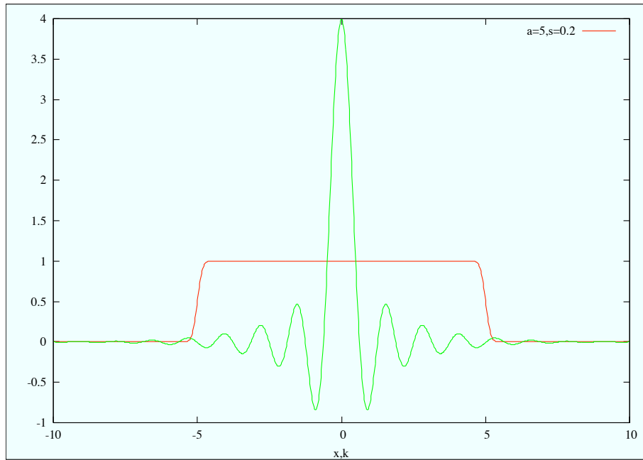
Figura 10: La funzione smoothed top-hat e la sua trasformata di Fourier
